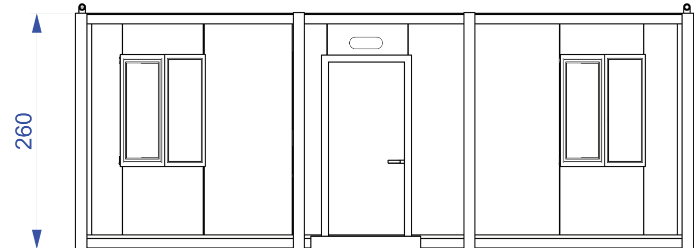
ÖN GÖRÜNÜŞ
